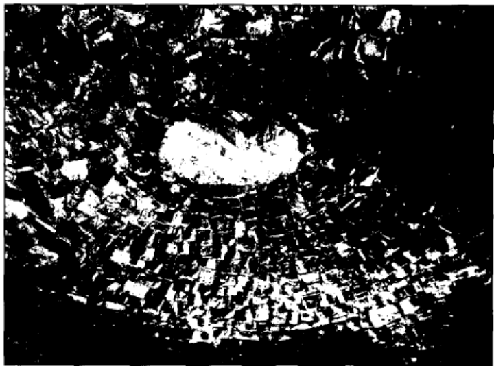
Vista de la cúpula i boca superior. Les llambordes són col·locades sense retocs de picapedrer. Observis a la part superior les sortint i cantelludes pedres de la fassa volta.
